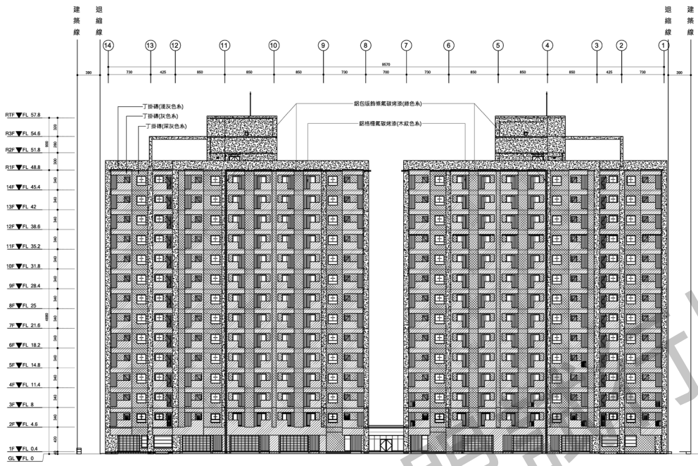
圖 2 北向立面圖
