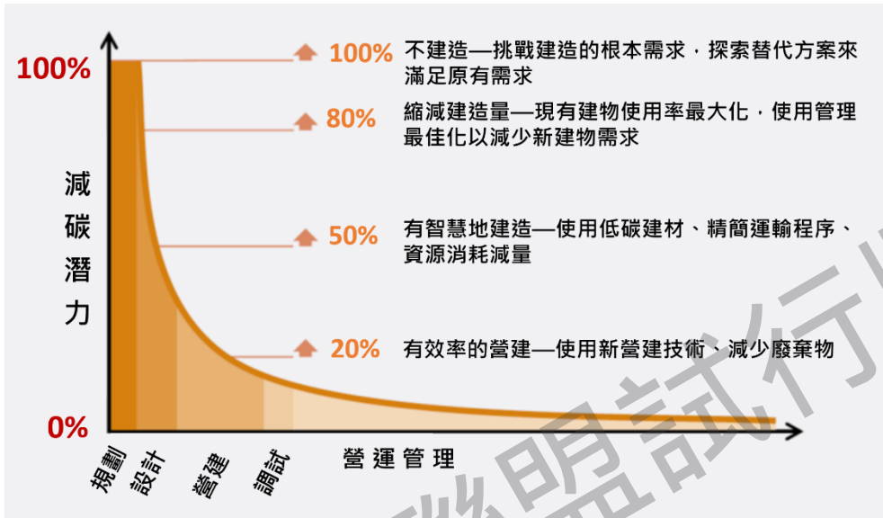
圖 11 建築蘊含碳排評估必須在設計階段執行快速評估、事前減碳方有最大減碳功能
