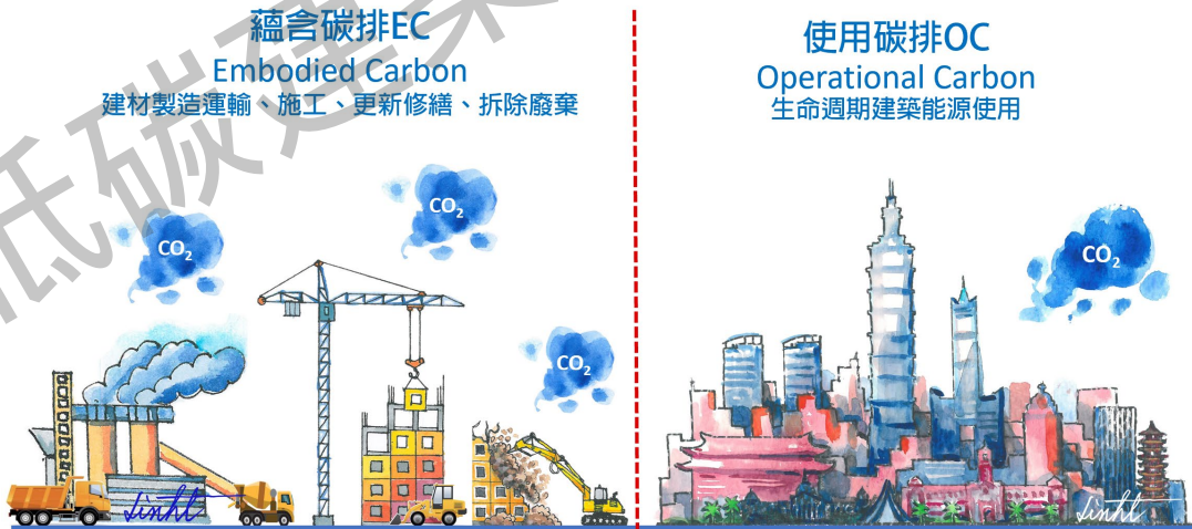
圖 3 全球建築物使用碳排 OC 與蘊含碳排 EC 在全球溫室氣體排放占比高達 28%與 9% (改繪自 IEA, 2022)
