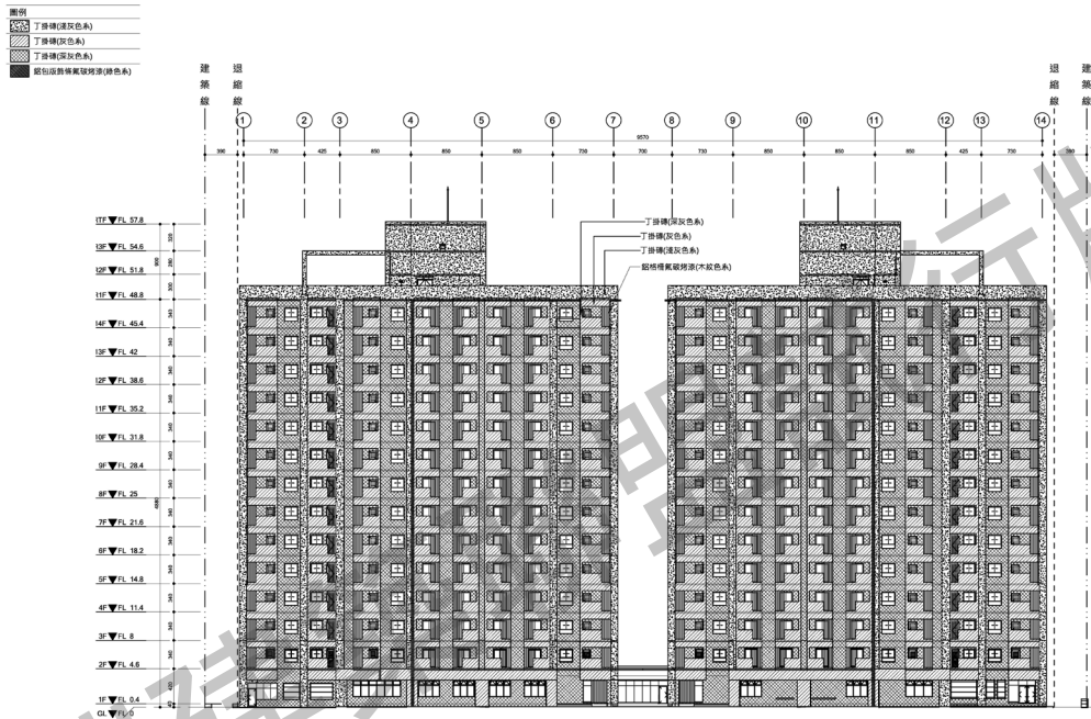
圖 1 南向立面圖
