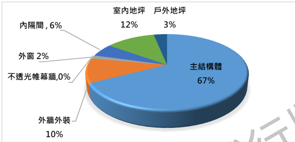
圖 11 設計案資材碳排佔比百分比圖（新建+修繕）
